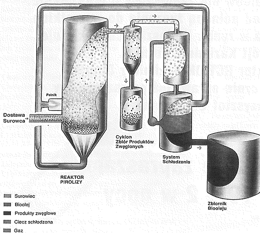
SCHEMAT PRODUKCJI BIOOLEJU TECHNOLOGIĄ SZYBKIEJ PIROLIZY.
