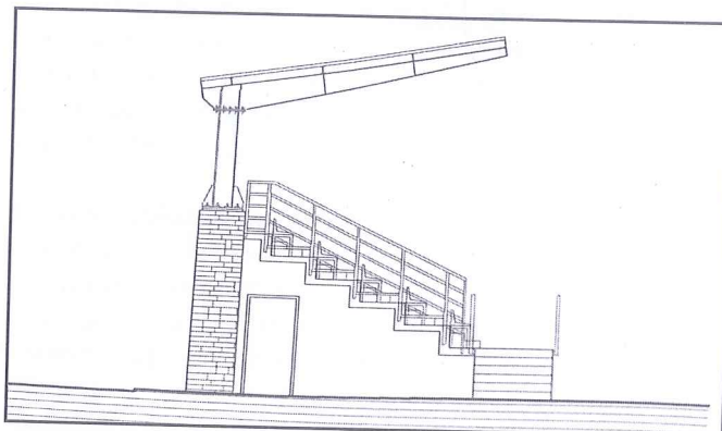
Projektowy przekrój trybuny.
