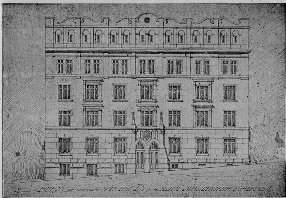
Projekt gmachu bursy dla dziewcząt T. S. L. we Lwowie.
