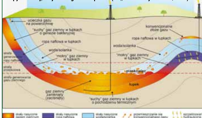
Uproszczony schemat występowania niekonwencjonalnych złóż gazu ziemnego i ropy naftowej, w tym złóż gazu w łupkach (za „Wiedza i Życie” Nr 2/2011).
